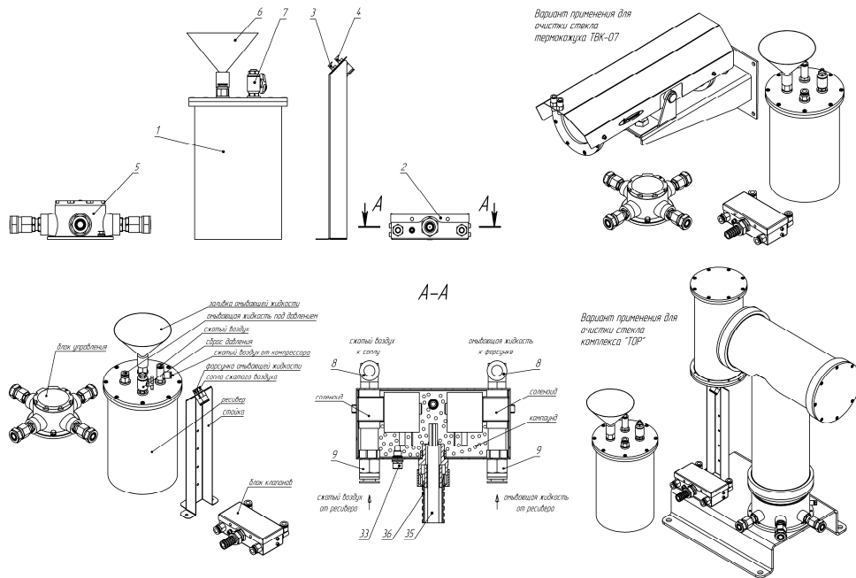
Рисунок 1. Функциональная схема системы очистки стекла.
