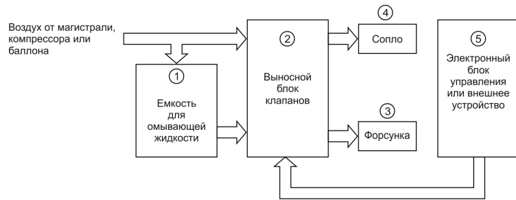
Рисунок 1. Функциональная схема системы очистки стекла.
